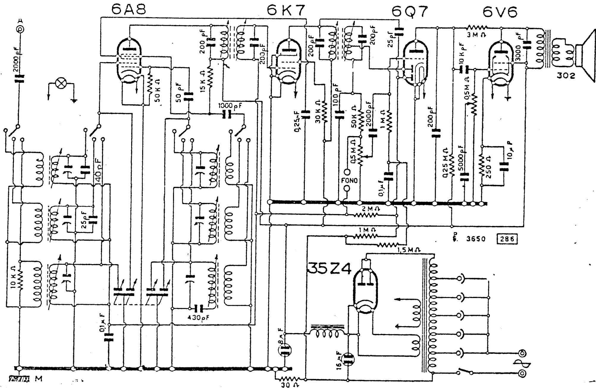
UNDA RADIO . MODD. « TRI UNDA '534' » « 538 »
